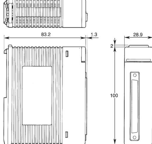
F3XD32
