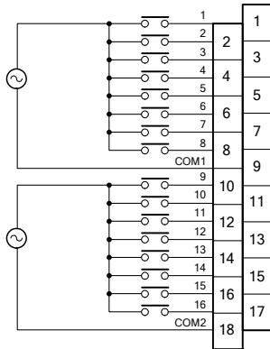
F3XA16-1N
