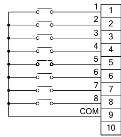
F3XC08-0N
