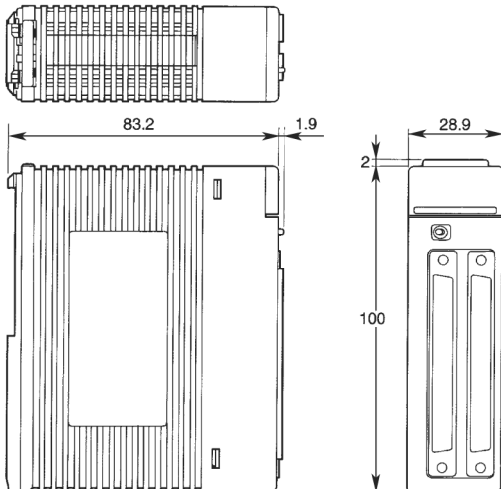
F3XD64-3F, F3XD64-4F
