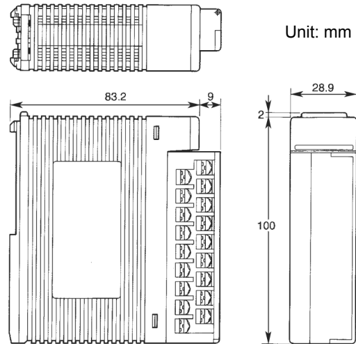
F3XC08-0C, F3XD16
