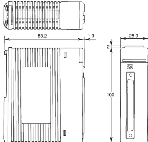
F3XD64-6M
