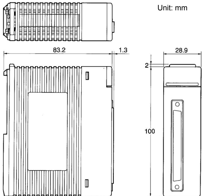
F3YD32-1H
