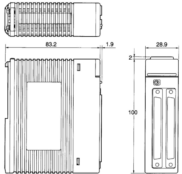
F3YD64-1P
