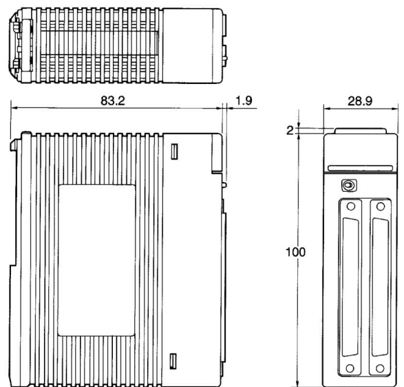
F3YD64-1R
