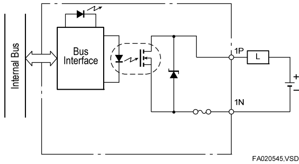
F3YD04-7N Transistor output module
