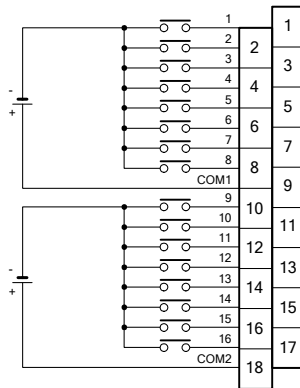
F3XD16-3H
