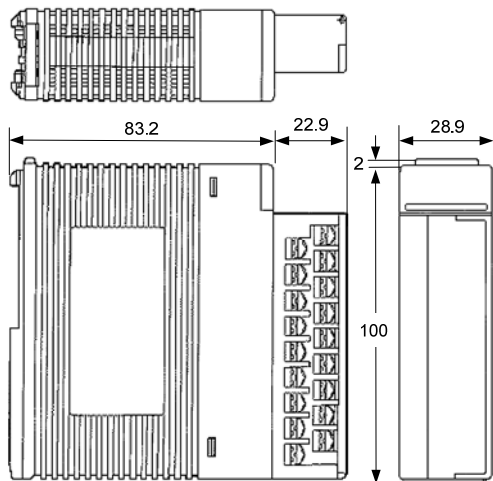
F3XA16
