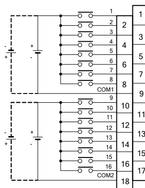
F3XD16-3F F3XD16-4F
